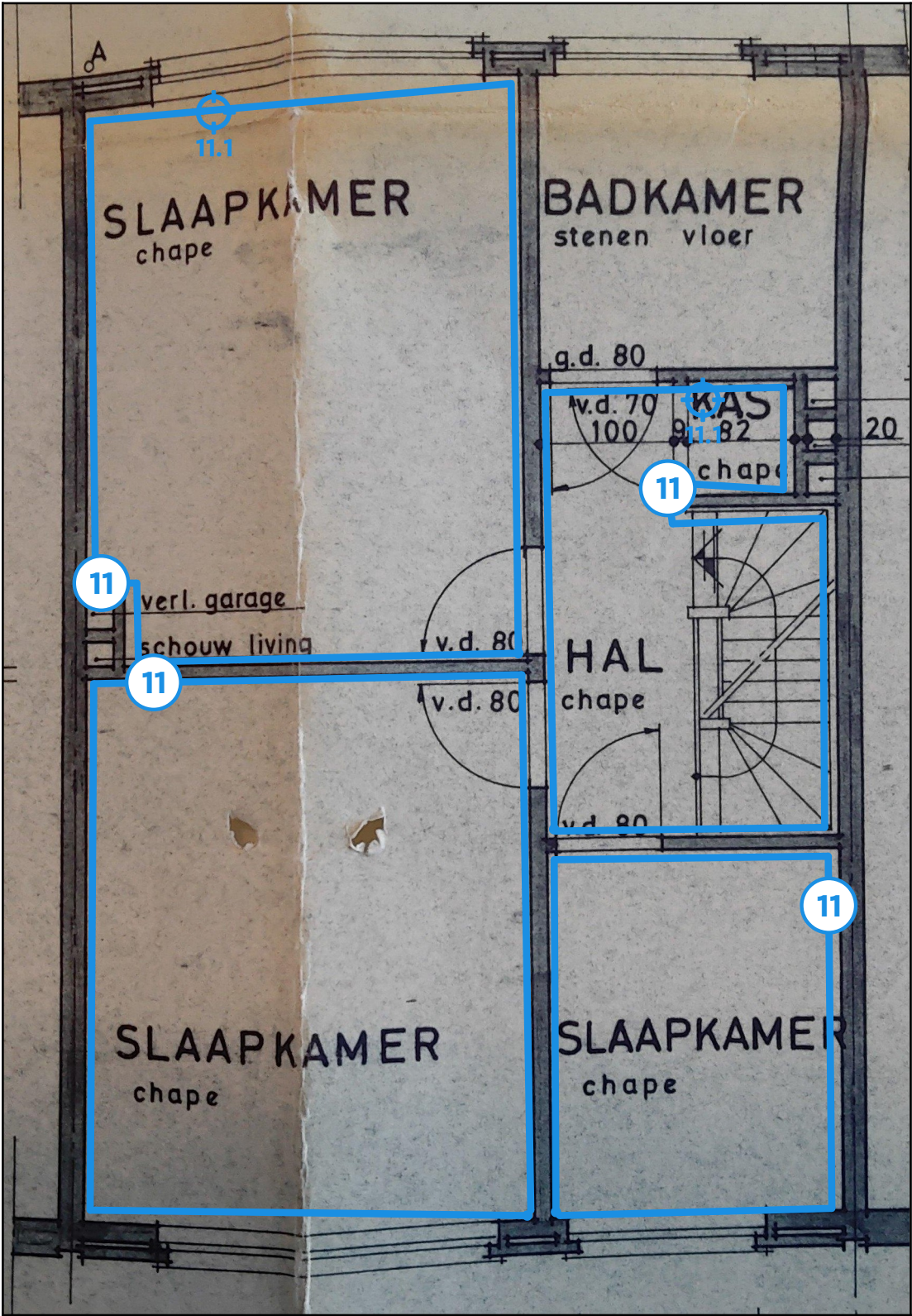
Legende van plan 1.8: Tweede verdieping
